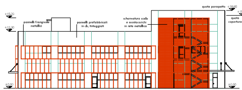
PROSPETTO NORD-EST
