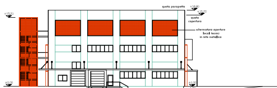
PROSPETTO NORD-OVEST
