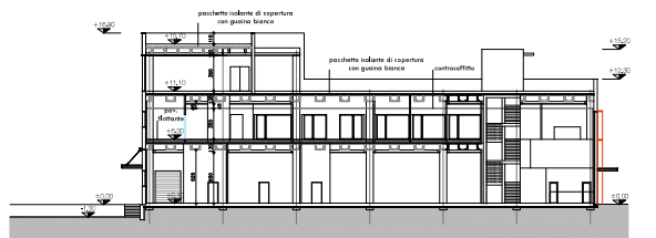
SEZIONE A - A1
