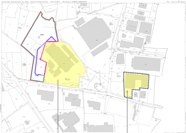
MAPPA CATASTALE 1:2.000
